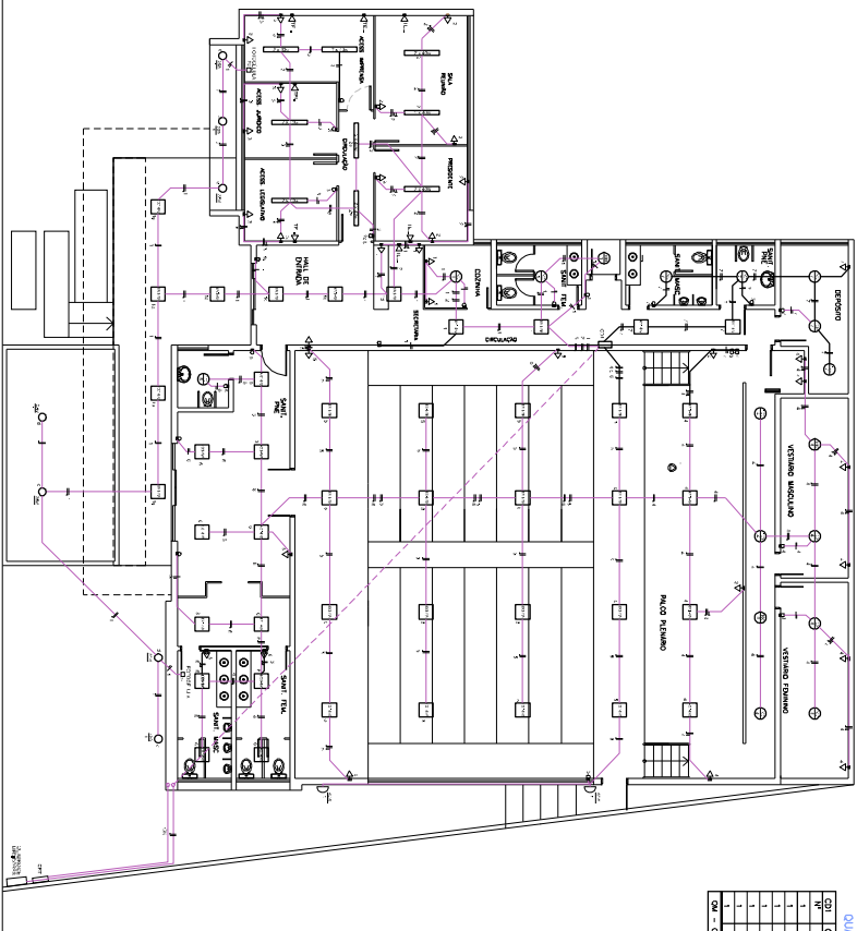
INSTALAÇÃO ELÉTRICA, escola: 1/75
