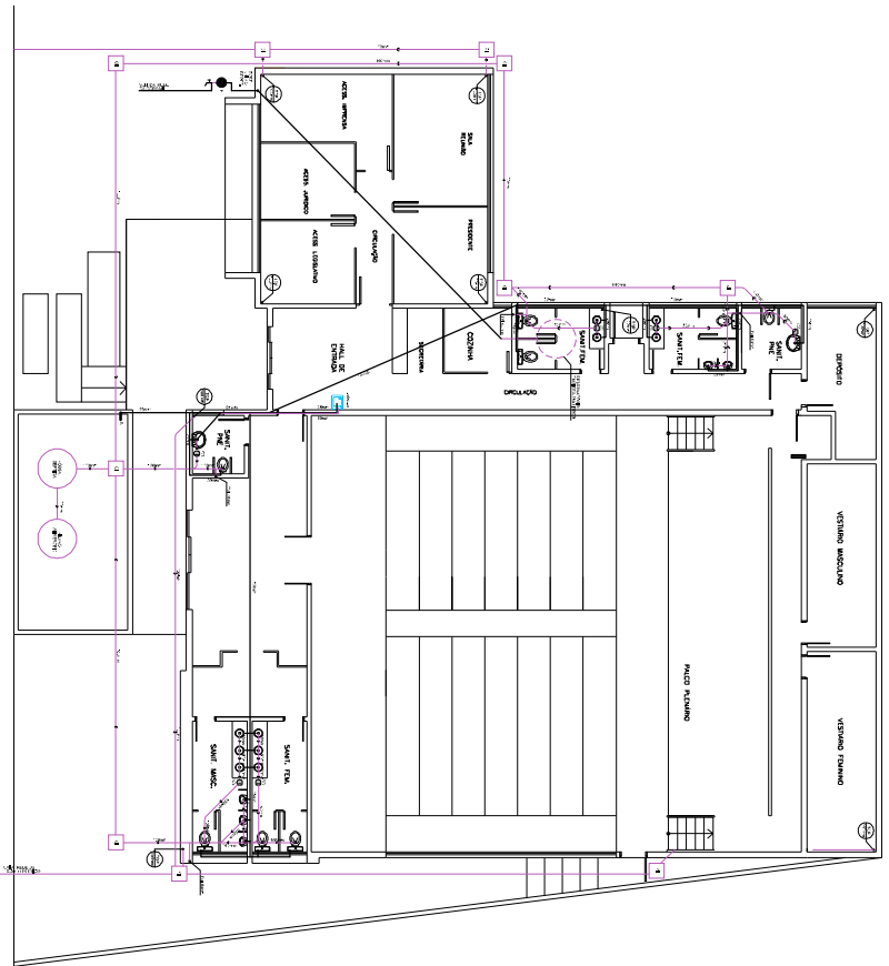
INSTALAÇÃO HIDROSSANITÁRIA, escada: 1/75 DETALHES DE INSTALAÇÃO
